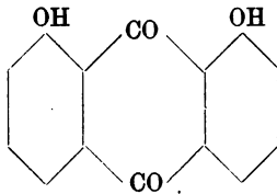
Chrysazin.
